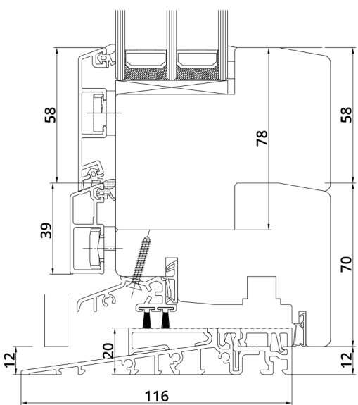
IDEALU CLASSICLINE IV 92 BALKONTÜRE MIT FLACHER SCHWELLE
