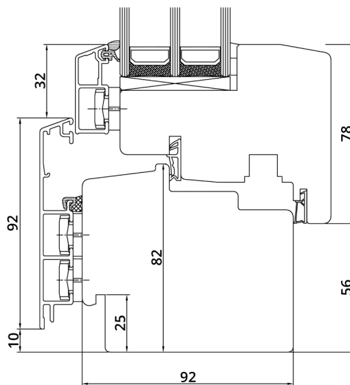
IDEALU CLASSICLINE IV 92 RAHMEN MIT FLÜGEL
